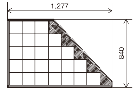
〈CS-124B61R 外形図〉
