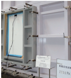
耐風圧試験の様子
