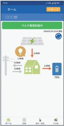
電力状況の確認 (リアルタイム)
