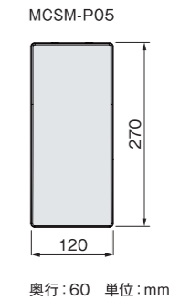
〈電力検出ユニット 外形図〉
