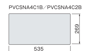
(昇圧回路付接続箱 外形図)
