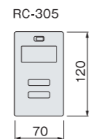
(リモコン 外形図)
