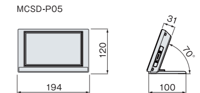
(カラーモニター 外形図)
