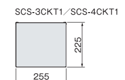
(接続箱 外形図)
