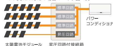
太陽電池モジュール 昇圧回路付接続箱
